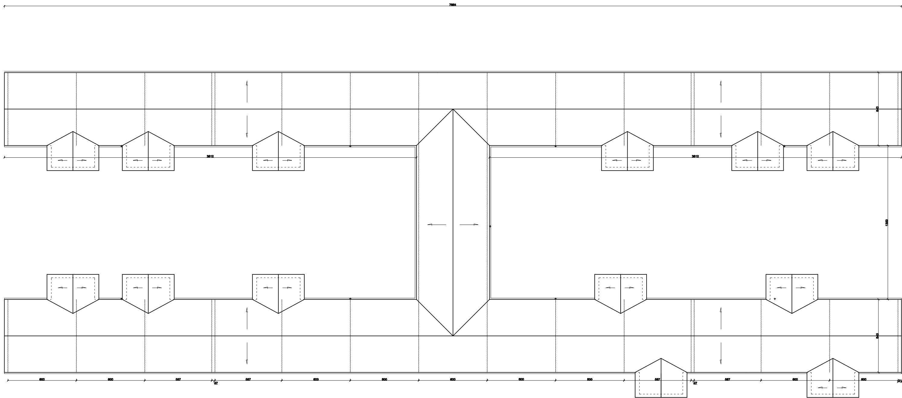
RZUT DACHU skala 1:100
