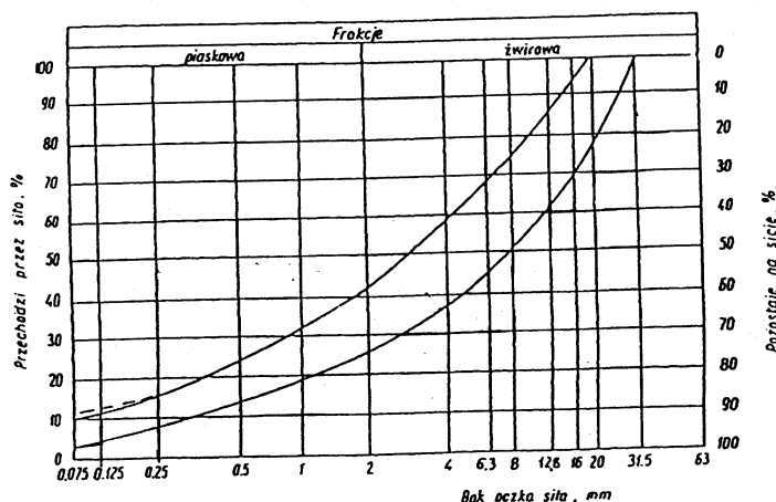
Rys. 1. Pole dobrego uziarnienia kruszywa dla podbudowy
