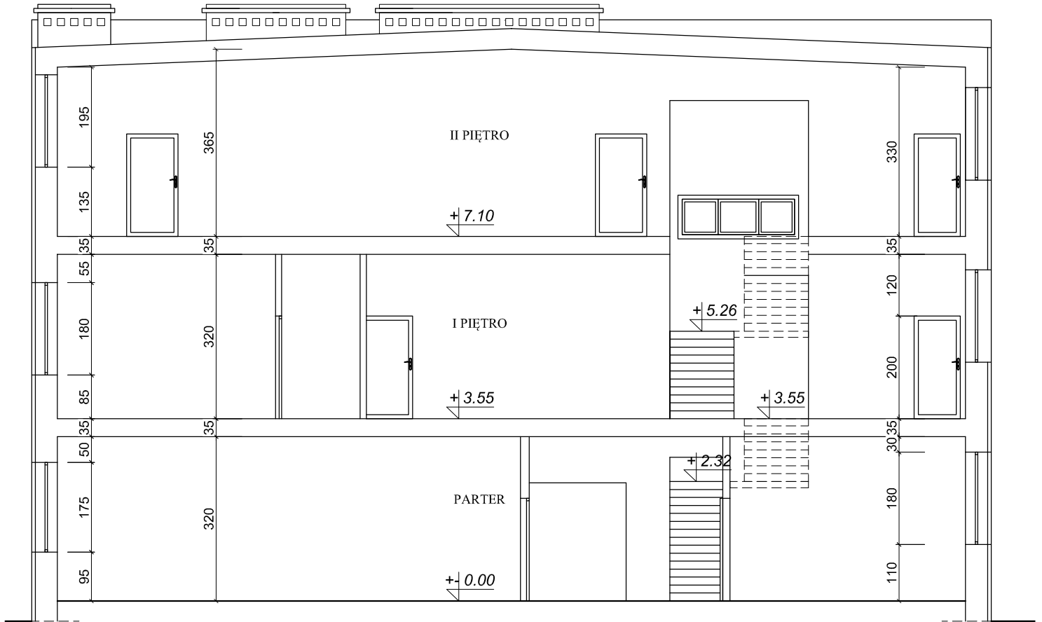
Przekrój A - A Stara szkoła
