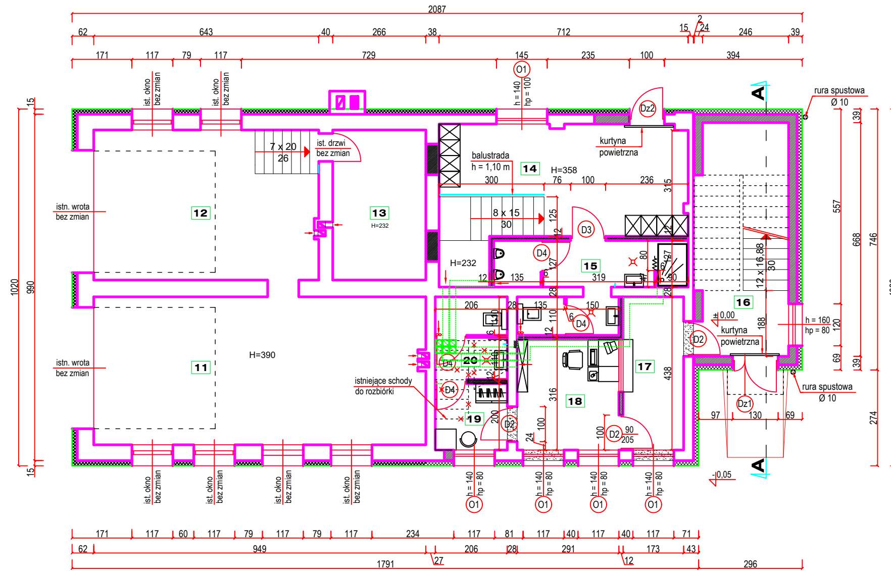
Rzut parteru 1 : 100
