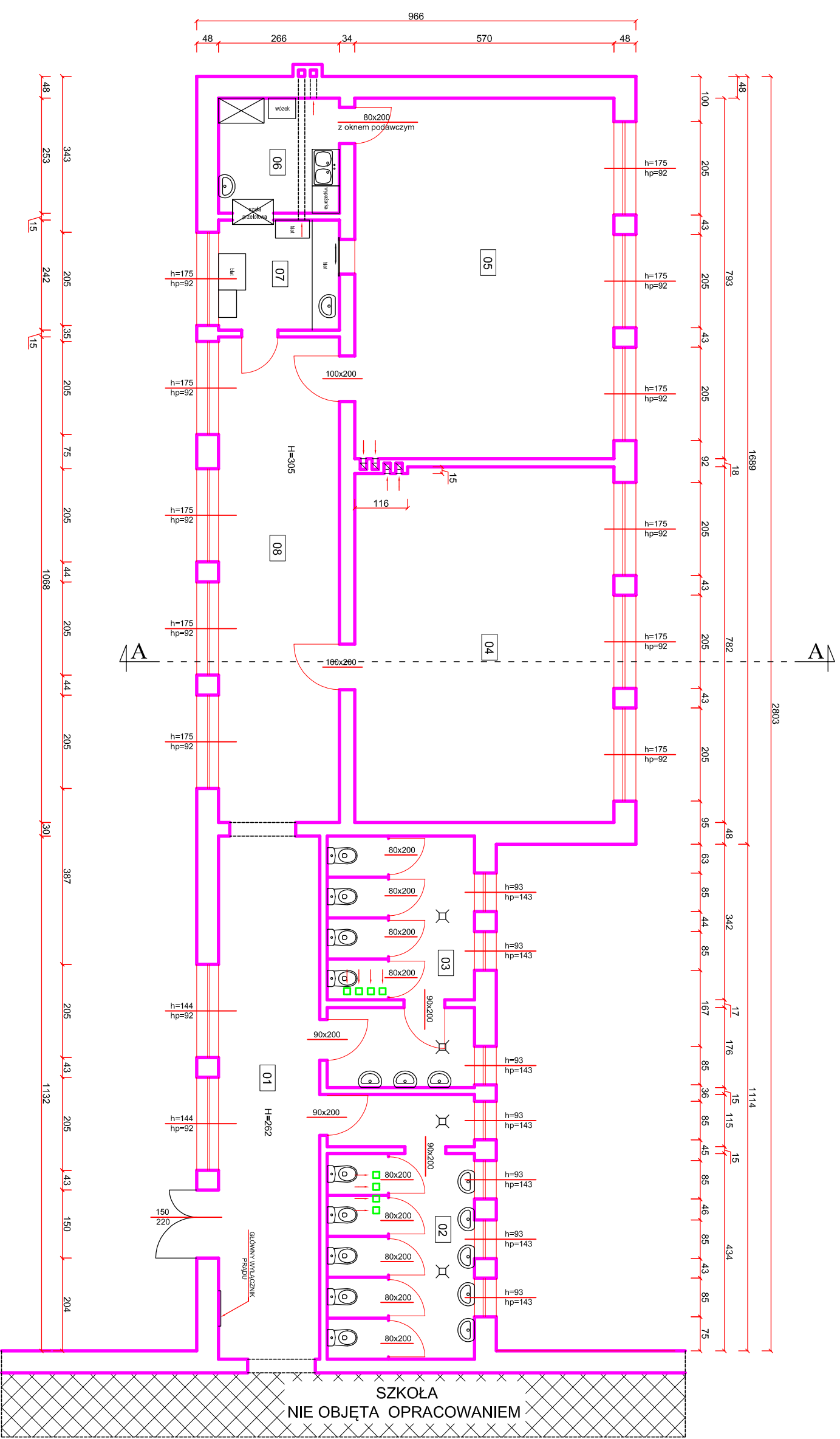
Rzut przyziemia 1: 100
