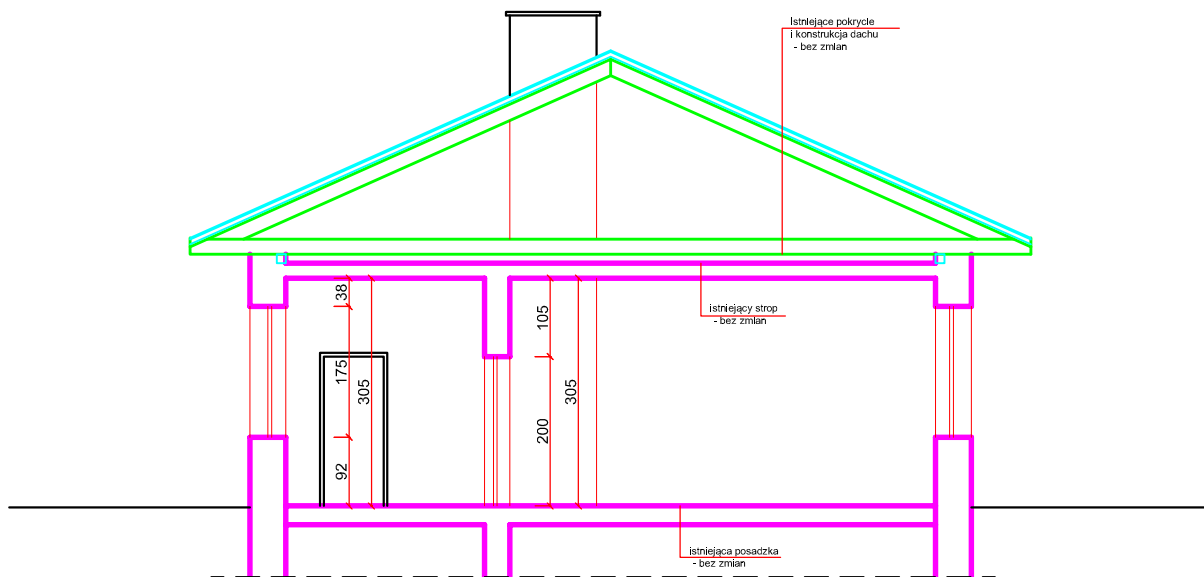
Przekrój A - A 1: 100
